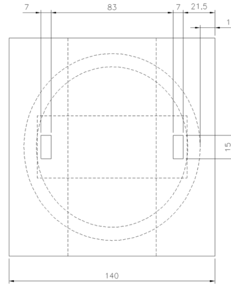
VISTA POSTERIOR LAMINILLA DE ANCLAJE Z-1561-0002r1
